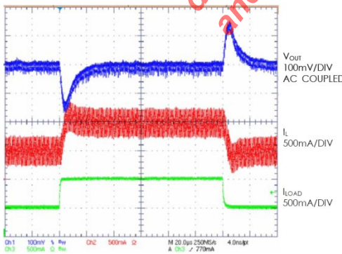
Fig. 20: Load Step
