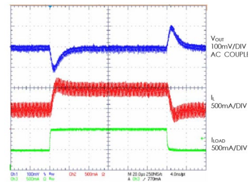
Fig. 21: Load Step
